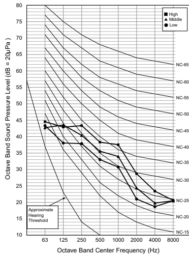
ARNU48GTAA4
