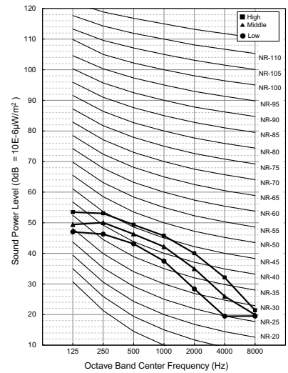
ARNU36GTAA4
