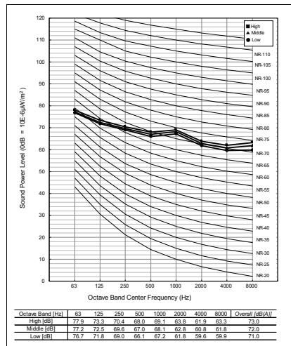
ARNU36GM2A4
