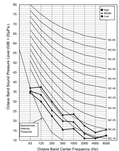
ARNU09GL4G4
