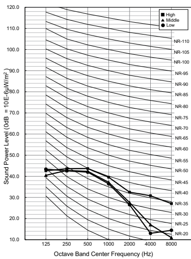
ARNU05GSJR4
