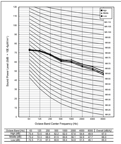
ARNU28GM2A4
