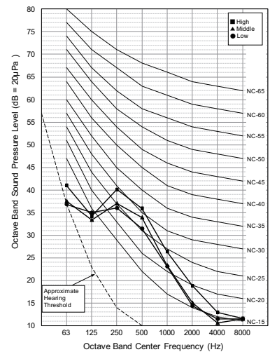
ARNU18GTS*4
