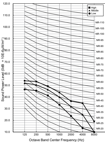
ARNU24GTS*4
