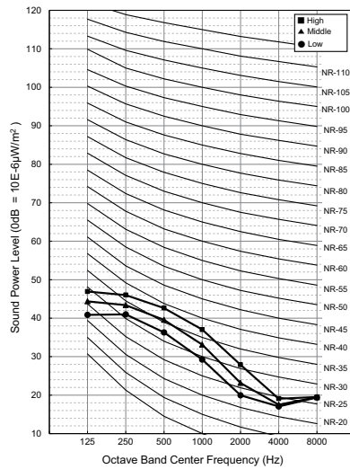
ARNU28GTAA4
