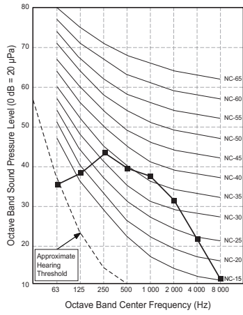
ARNU18GTT*4
