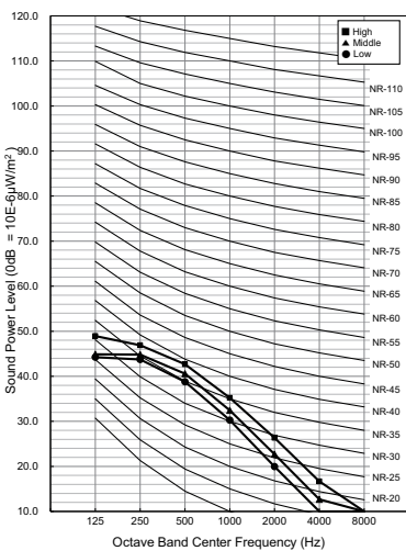
ARNU24GTS*4
