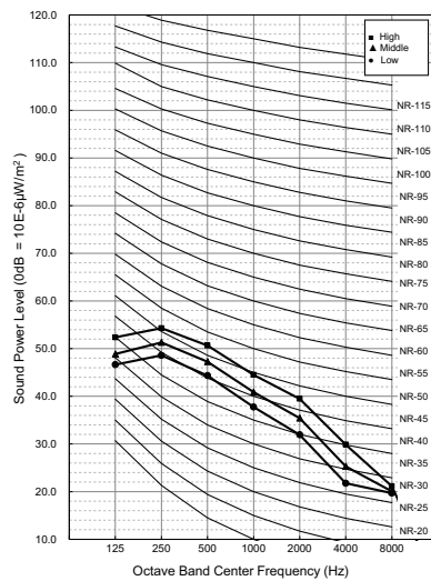
ARNU36GTYA4
