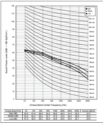
ARNU28GM2A4
