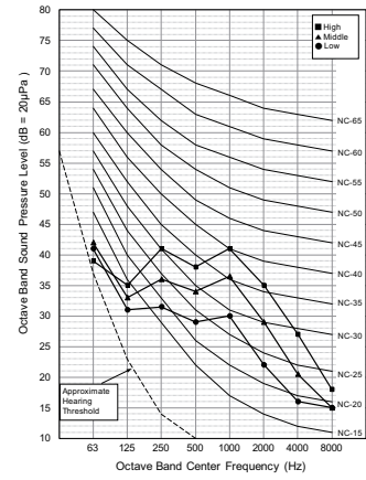
ARNU36GSVA4
