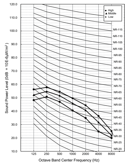
ARNU48GTYA4
