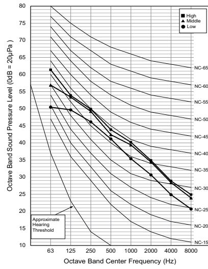
ARNU36GM2A4
