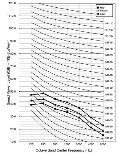
ARNU09GL4G4
