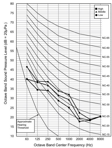
ARNU36GTAA4
