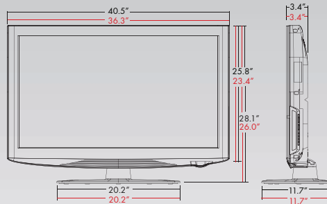
32LH200C
